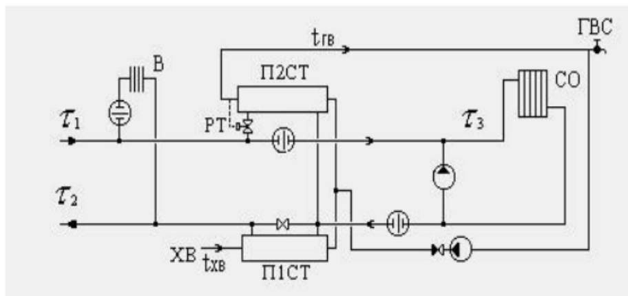
Рисунок 15. Принципиальная 2-ступенчатая схема включения теплообменников ГВС в ИТП
